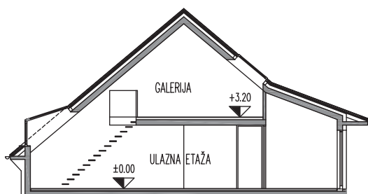
SHEMATSKI PRESJEK
