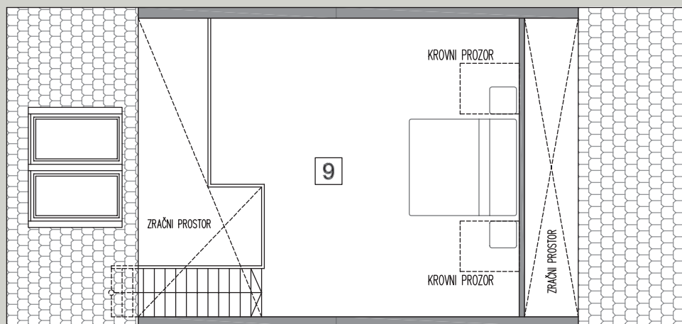
TLOCRT GALERIJE
