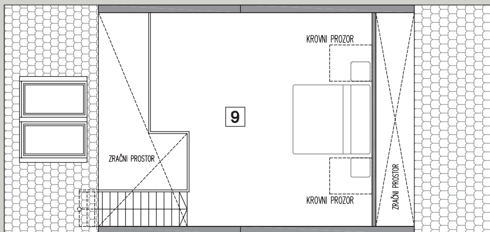
TLOCRT GALERIJE
