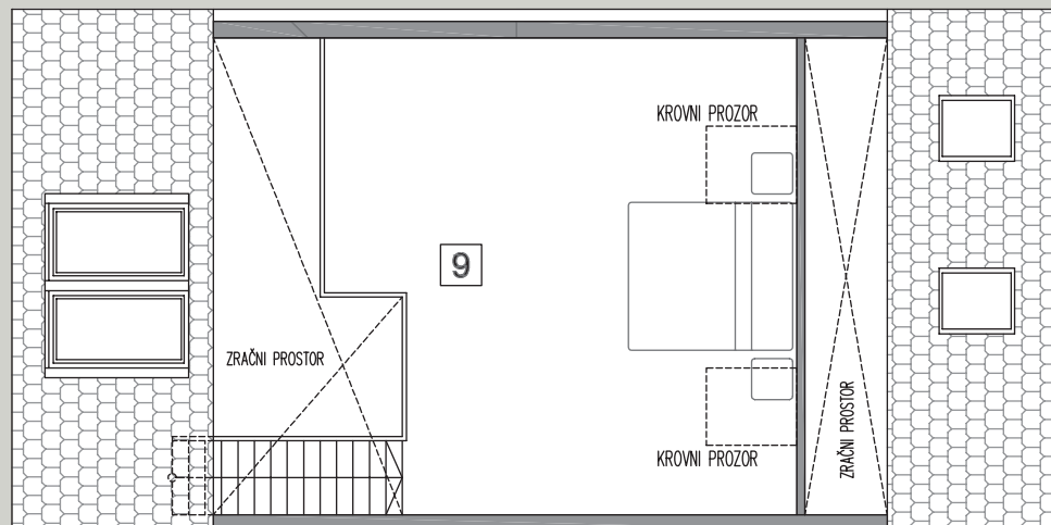
TLOCRT GALERIJE
