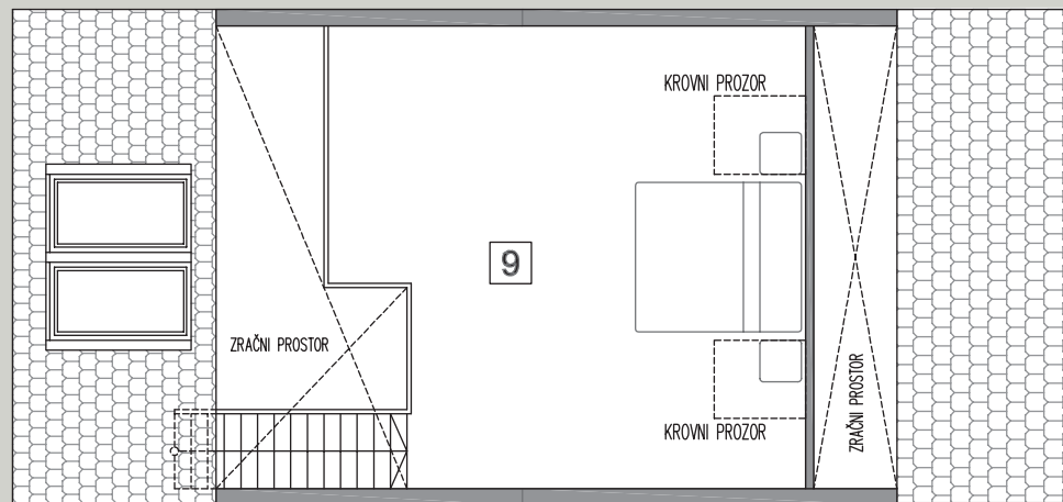
TLOCRT GALERIJE
