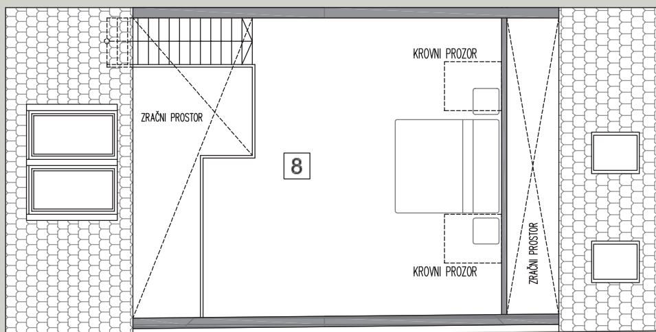
TLOCRT GALERIJE
